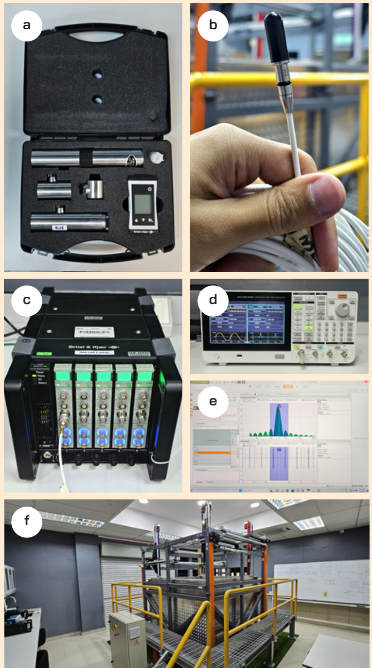
Rajah 1: Fasiliti dan perkakasan yang digunakan dalam pengujian akustik bawah air (a) Kalibrator transduser, (b) Transduser 8103 dengan kabel integral, (c) Data Acquisition System (DAQ) (d) Penjana isyarat, (e) Perisian BK Connect@ dan (f) Kolam akustik
